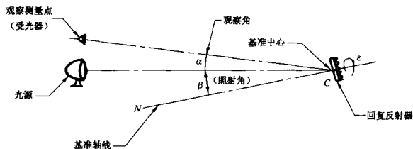
图 1 光度测试原理图
